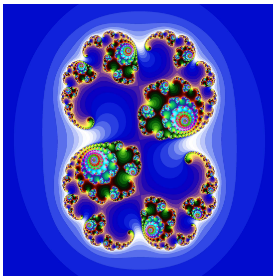
FIGURE 7 – L'ensemble de Julia, dont le contour est un courbe sans tangentes
