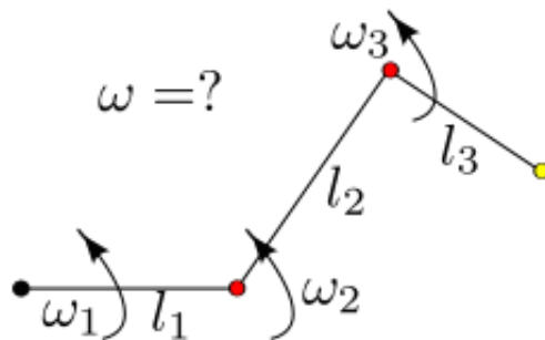
FIGURE 4 – Le problème de Lagrange consiste à étudier le mouvement du bras articulé. Ce bras consiste en N segments de longueurs l_1, \dots, l_N \in \mathbb{R}_+ , attachés en une chaîne. Chacun des segments tourne avec une vitesse angulaire constante \omega_j, j = 1, \dots, N autour de l'extrémité du segment précédent. L'intérêt de Lagrange se portait sur la vitesse angulaire asymptotique \omega de l'extrémité de ce système, définie comme la limite \frac{N(T)}{T} où N(T) est le nombre de tours effectués en temps T . Lagrange voulait prouver l'existence de cette limite et trouver son expression en terme des longueurs l_j et des vitesses angulaires \omega_j .
