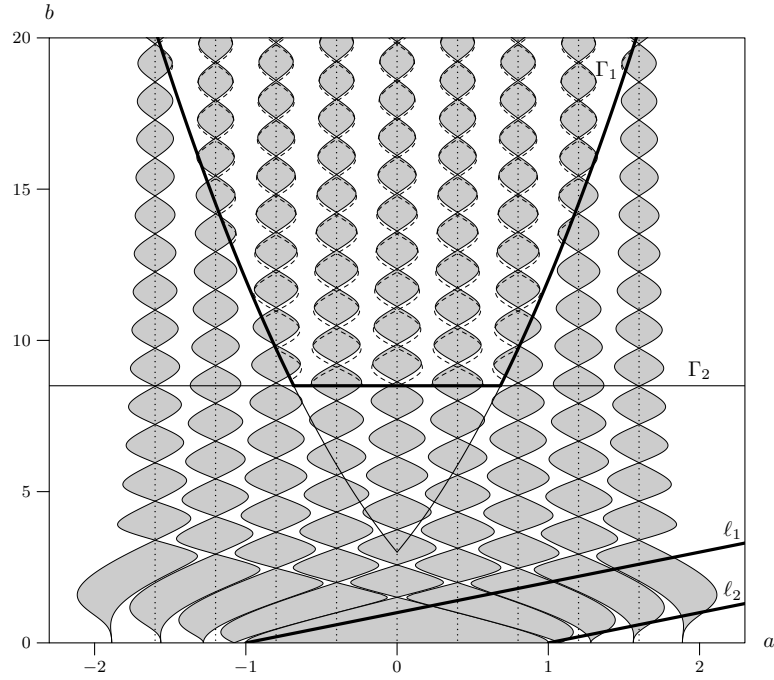
FIGURE 3 – L'image représentant les sections des langues d'Arnold de l'équation de Josephson (1) à \mu fixé, \mu = 0.4 . Les langues représentées correspondent aux valeurs entières du nombre de rotation \bar{\rho} = -4, \dots, 4 . Dans la première partie du chapitre 1 nous démontrons la proximité des frontières des langues et des fonctions entières de Bessel quand b \rightarrow \infty : notre preuve fonctionne dans une zone au-dessus des courbes \Gamma_1 et \Gamma_2 , définies plus précisément au cours du chapitre 1. Les frontières de cette zone sont marquées en gras, et les graphes des fonctions de Bessel en pointillés. Dans la deuxième partie du chapitre 1 nous étudions un autre régime limite : \mu \rightarrow 0 , qui est plus pertinent du point de vue physique. La zone étudiée dans ce régime est la zone entre deux droites \ell_1 et \ell_2 ainsi que la zone bornée au-dessus de la droite \ell_1 . Nous prouvons la proximité des langues au sein de ces deux zones quand \mu \rightarrow 0 ; déjà sur ce dessin nous pouvons voir que les langues sont très proches autour de la droite \ell_1 .
