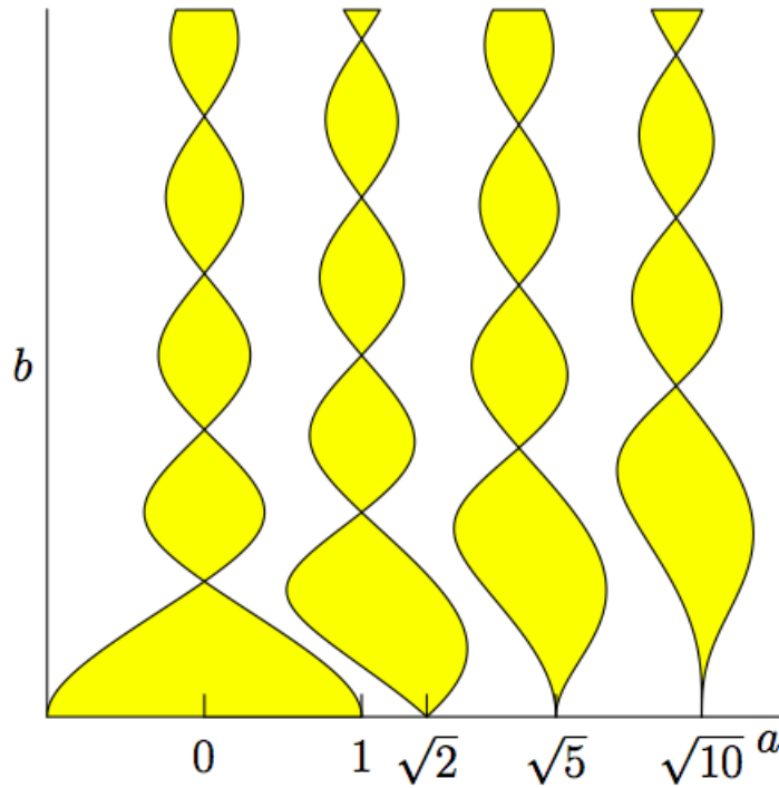
FIGURE 2 – La structure géométrique des langues d’Arnold pour l’équation de Josephson (1) est assez originale par rapport au dessin correspondant à la famille standard d’Arnold, voir Figure 1 : les frontières des langues s’auto-intersectent en formant des « tresses ». Ici sont dessinées les sections des langues avec un plan \{\mu = 1\} . L’image représente les sections des langues (sur le plan (a, b) \in \mathbb{R}^2 ) correspondant aux valeurs entières du nombre de rotation : \bar{\rho} = 0, 1, 2, 3 . Notons que la langue d’Arnold correspondant à \rho = 0 contient tout le segment [-1, 1] \times 0 (l’équation correspondante a une solution constante). Les sections des langues correspondant à \bar{\rho} = k \in \mathbb{Z} « commencent » aux points \sqrt{1 + k^2} .
