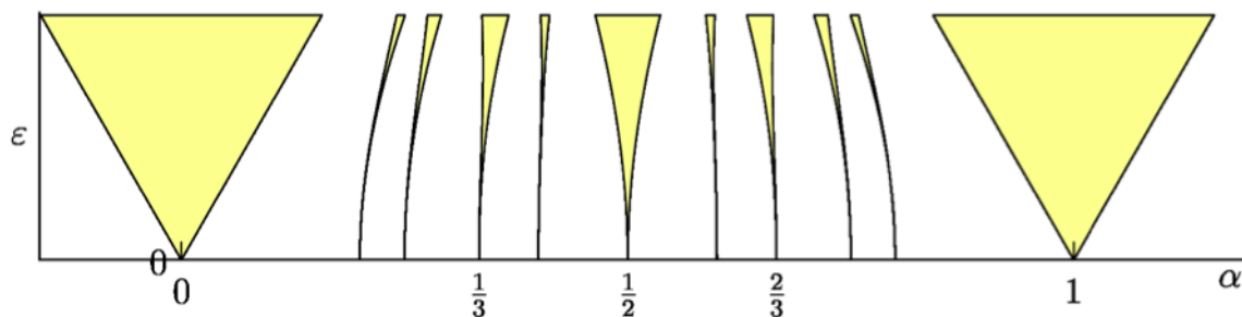
FIGURE 1 – L'ensemble des langues d'Arnold de la famille (3) pour toutes les valeurs du nombre de rotation \rho = \frac{p}{q} avec dénominateur q \leq 5 . Chaque langue a une « racine » au point (\frac{p}{q}, 0) correspondant à la rotation pure avant de grossir petit à petit avec \varepsilon qui grandit. Pour cette famille, les langues d'Arnold existent pour toutes les valeurs rationnelles de \rho = \frac{p}{q} et leur largeur diminue quand q augmente.
